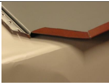
Färdig plåt vid vinkelrännans början
