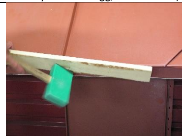
Montage av första plåt vid vinkelränna
